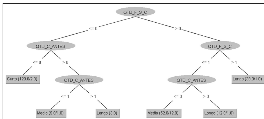
Figura 2 – Árvore de regras gerada pela análise do J48 da fase 1 da Atividade 1
