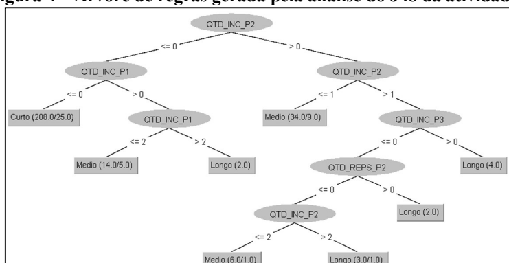
Figura 4 – Árvore de regras gerada pela análise do J48 da atividade 4
