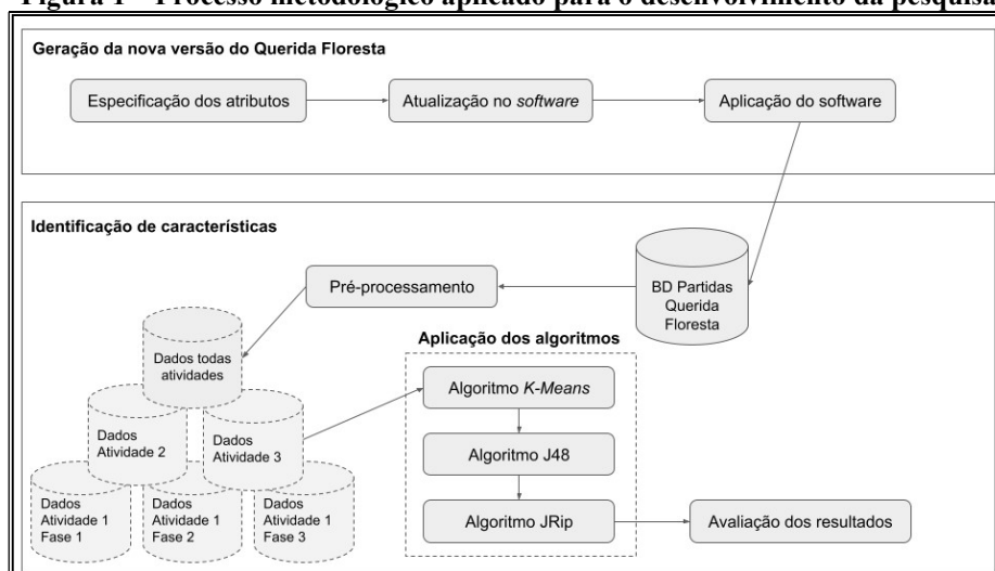
Figura 1 – Processo metodológico aplicado para o desenvolvimento da pesquisa
