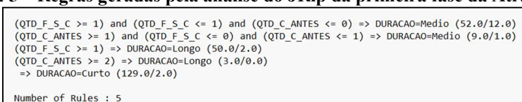
Figura 5 – Regras geradas pela análise do JRip da primeira fase da Atividade 1
