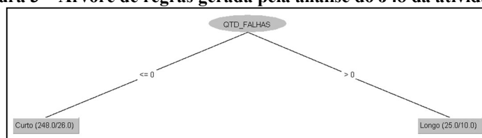
Figura 3 – Árvore de regras gerada pela análise do J48 da atividade 2
