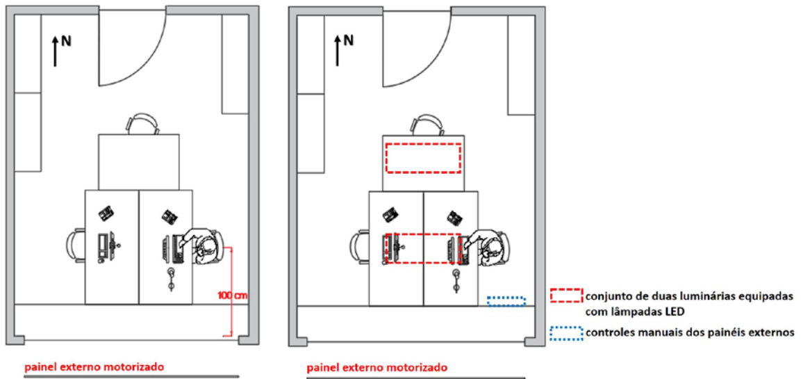
Figura 7 - (a) Posição ocupada pelo usuário durante o experimento; e (b) Localização dos controles manuais e da iluminação artificial
