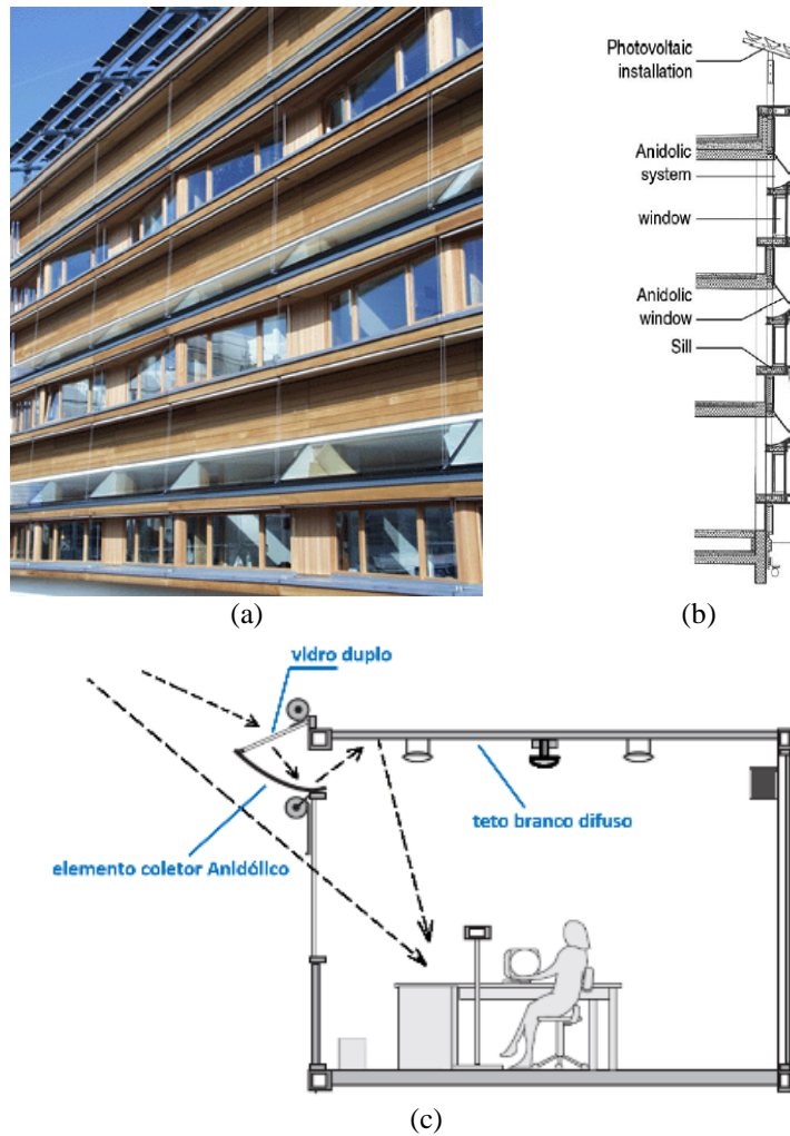
Figura 8 - (a) ADS na fachada sul; (b) Seção transversal na fachada sul; e (c) Vista esquemática da sala LE001 equipada com ADS
