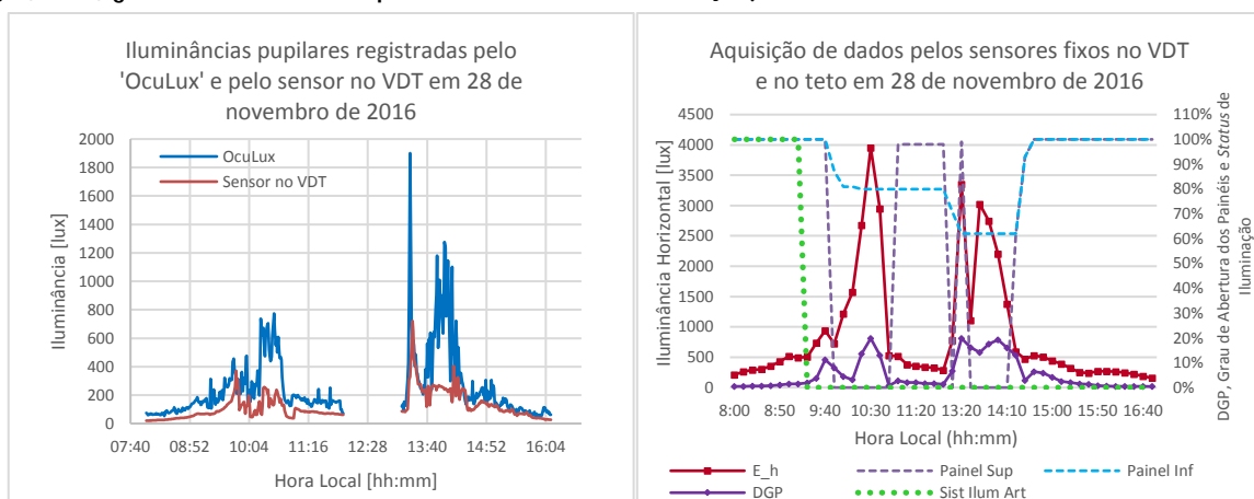
Figura 13 - Dados para 28 de novembro de 2016 sob céu parcialmente encoberto: (a) Registro das iluminâncias pelo "OcuLux" e pelo sensor fixado no VDT; e (b) Aquisição de dados pelos sensores fixos ( E_h , DGP, grau de abertura dos painéis e status de iluminação)
