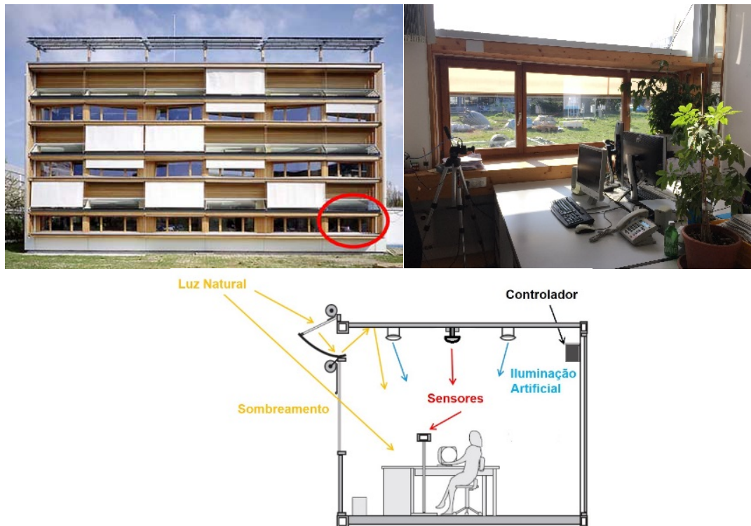
Figura 5 - (a) Fachada Sul do LESO-PB. Em destaque a sala LE001 onde o experimento foi realizado; (b) Interior da sala; e (c) Localização usual dos sensores
