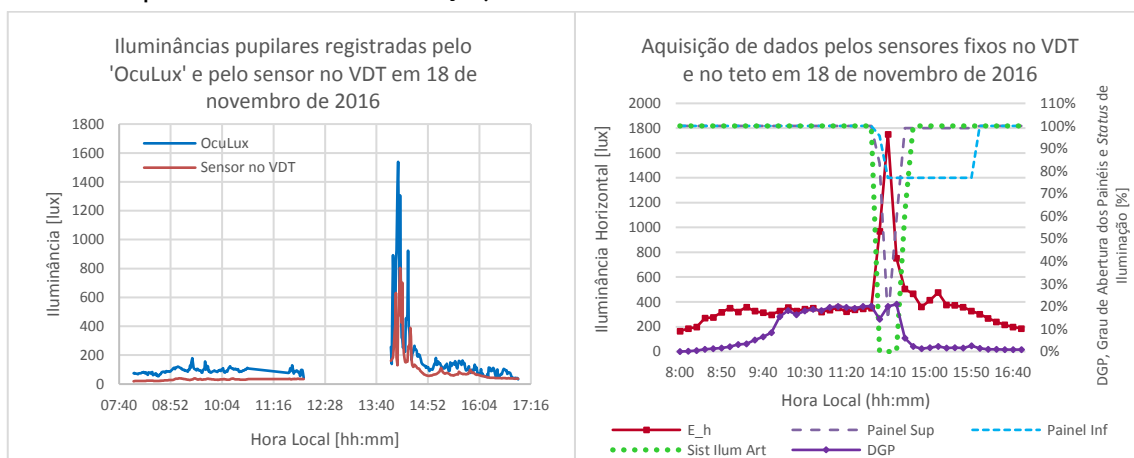
Figura 12 - Dados para 18 de novembro de 2016 sob céu encoberto: (a) Registro das iluminâncias pelo “OcuLux” e pelo sensor fixado no VDT; e (b) Aquisição de dados pelos sensores fixos ( E_h , DGP, grau de abertura dos painéis e status de iluminação)
