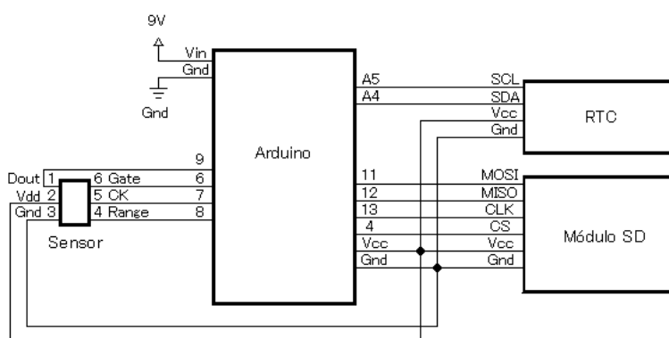
Figura 11 - Diagrama eletrônico do “OcuLux”
