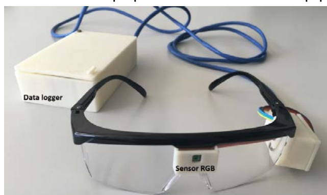
Figura 10 - Dispositivo vestível “OcuLux” que permite avaliar a iluminância pupilar (lux) em tempo real
