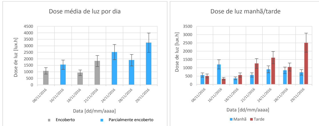
Figura 14 - (a) Dose média de luz [lux.h] recebida pelo usuário durante o experimento; (b) Dose de luz [lux.h] recebida por período
