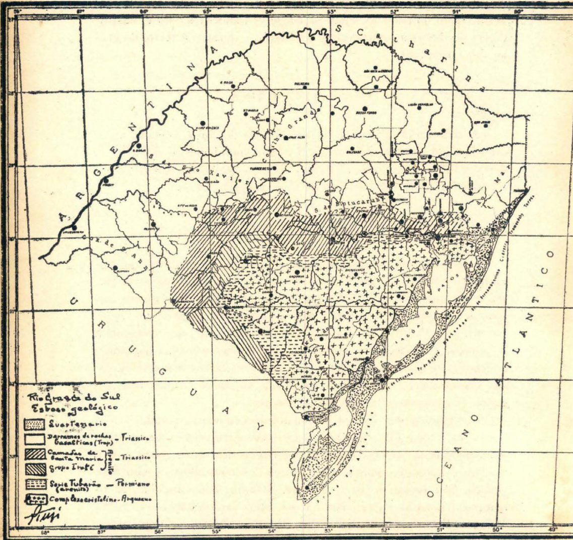
Esboço geológico do Rio Grande do Sul
