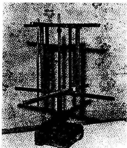
Dobadoira (também conhecida por argadilho ou debanadeira)
