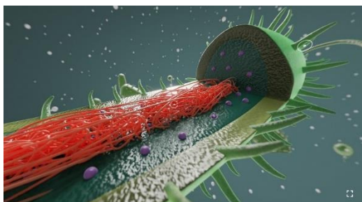
Figura 2 – Célula procariótica
