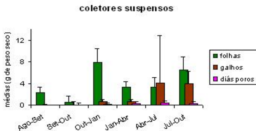
Figura 2. Contribuição das partes vegetativas (folhas e galhos) e reprodutivas (diásporos) em coletores suspensos para cada período de coleta, no período de Agosto/2004 a Outubro/2005 na nascente do riacho Garapiá, São Francisco do Sul, RS.
