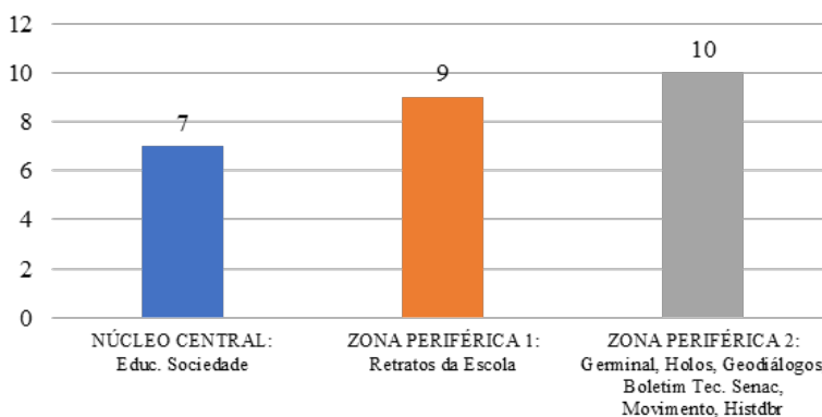
Gráfico 1 - Classificação dos Periódicos
