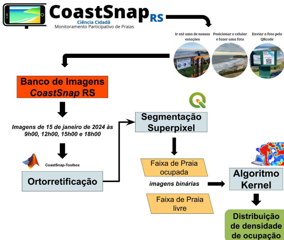
Figura 3 - Fluxograma metodológico.
