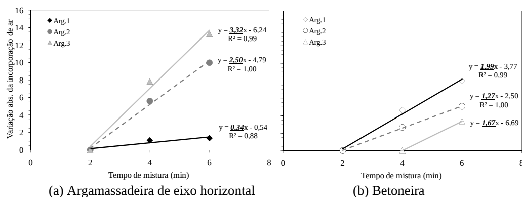
Figura 5 - Variações nos teores de ar absolutos em função da mistura por 2 min
