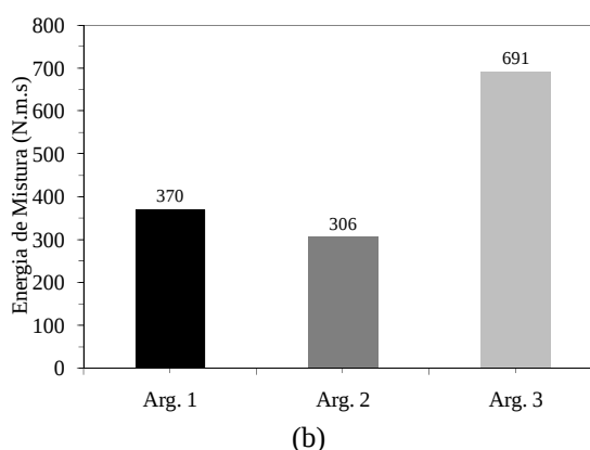
Figura 6 - Curvas de mistura das argamassas (a) e estimativas das energias de mistura (b), calculadas a partir das áreas abaixo das linhas do gráfico de torque vs tempo
