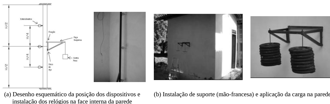
Figura 5 - Ensaio de cargas provenientes de peças suspensas em parede do protótipo
