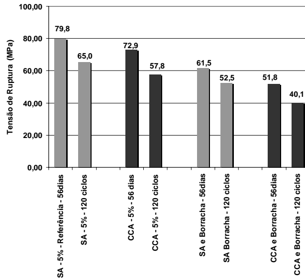
Figura 10 - Comparação da resistência à compressão antes e após o ensaio
