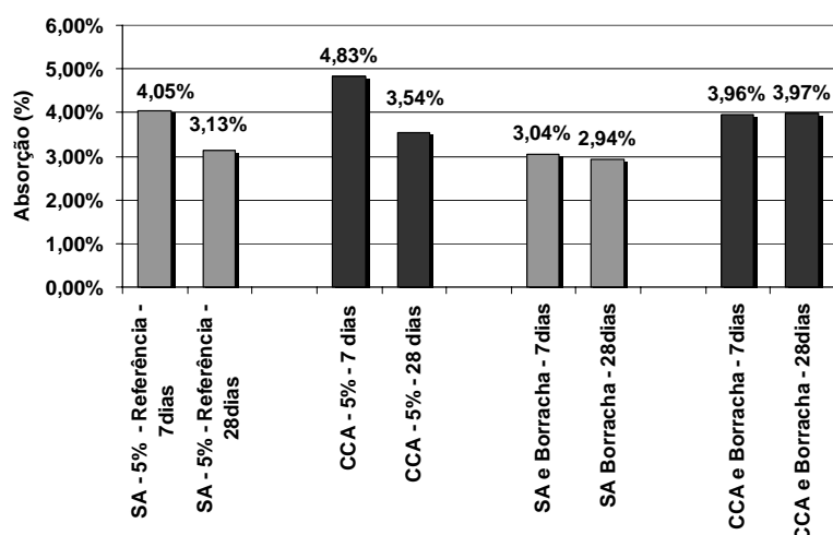
Figura 7 - Absorção de água por imersão no concreto
