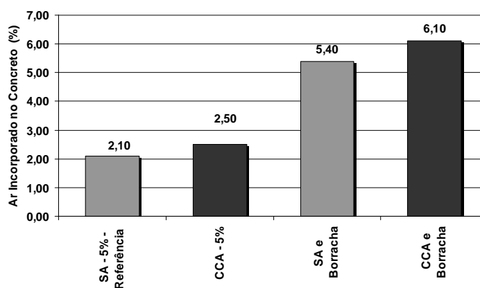
Figura 4 - Incorporação de ar no concreto
