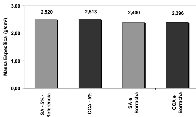
Figura 5 - Massa específica do concreto fresco
