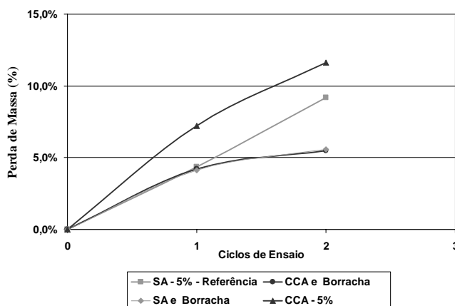
Figura 13 - Resultado da perda de massa após o ataque químico
