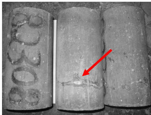
Figura 11 - Aparecimento de eflorescência
