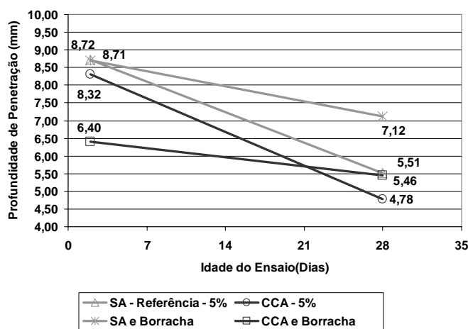
Figura 9 - Penetração de água sob pressão
