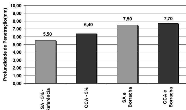
Figura 14 - Profundidade de penetração de cloretos
