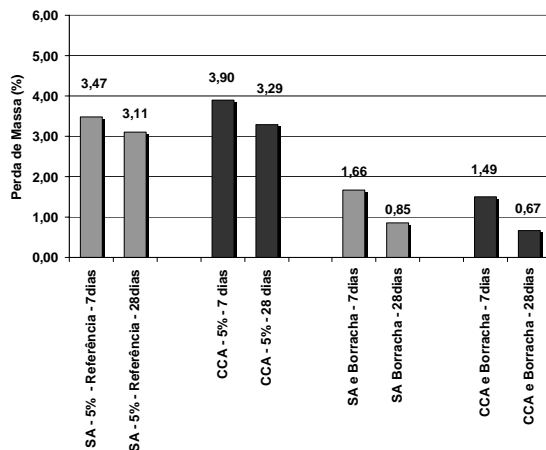
Figura 15 - Perda de massa por abrasão/erosão
