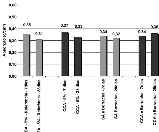
Figura 8 - Absorção de água por capilaridade no concreto
