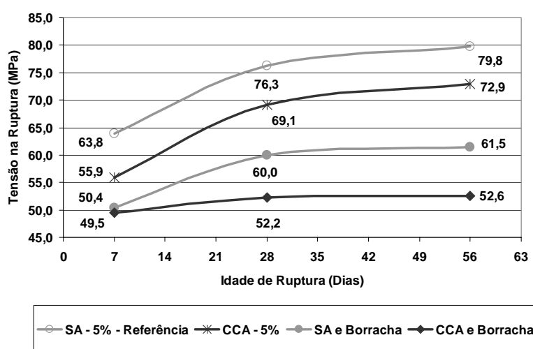
Figura 6 - Resistência à compressão dos traços estudados
