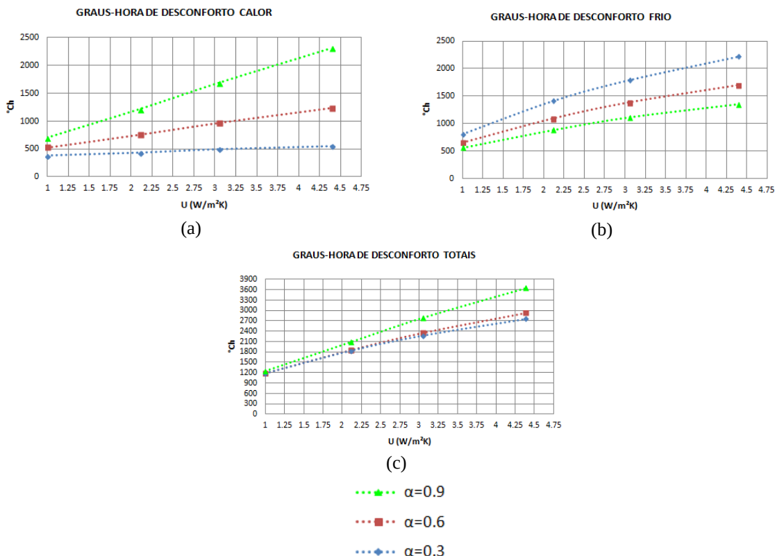
Figura 5 - Graus-hora de desconforto totais anuais para a habitação, com variados U e \alpha das paredes, U_{\text{cobertura}}=1,8 \text{ W/m}^2 \text{ K} e \alpha_{\text{cobertura}}=0,9 , em São Paulo
