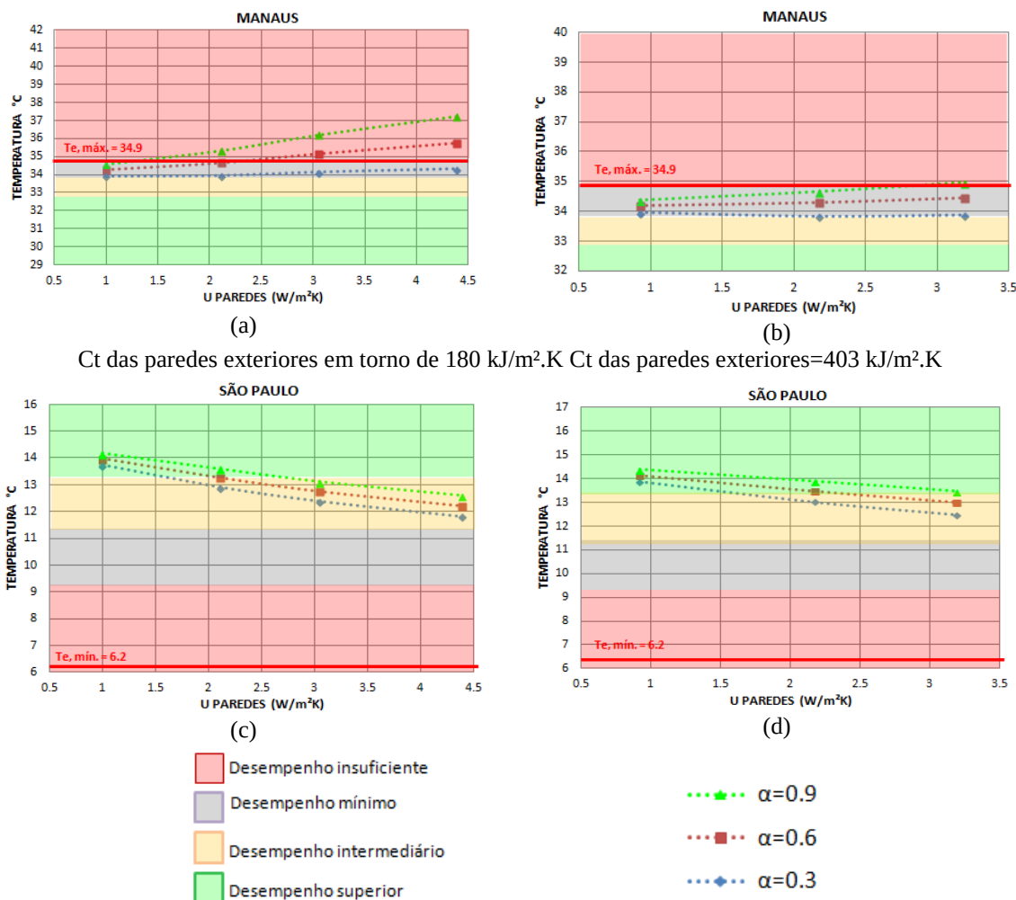
Figura 4 - Habitação com variados U e \alpha das paredes, U_{\text{cobertura}}=1,80 \text{ W/m}^2 \text{ K} e \alpha_{\text{cobertura}}=0,9
