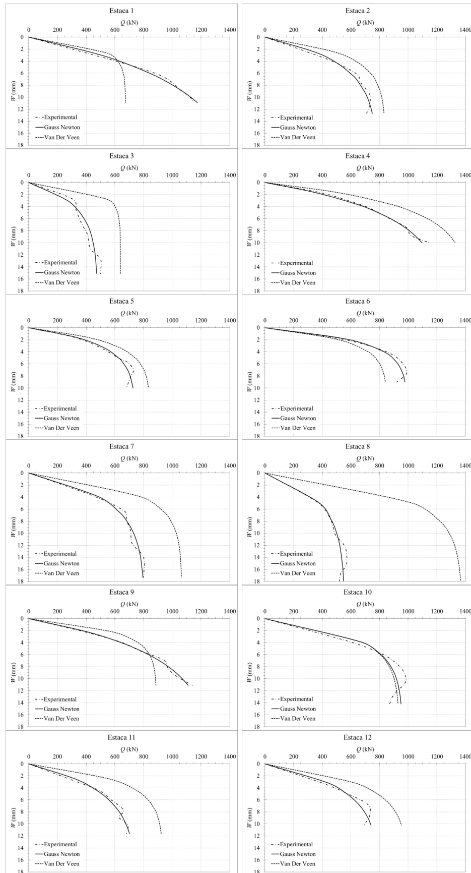
Figura 5 – Curvas carga-recalque das estacas de madeira
