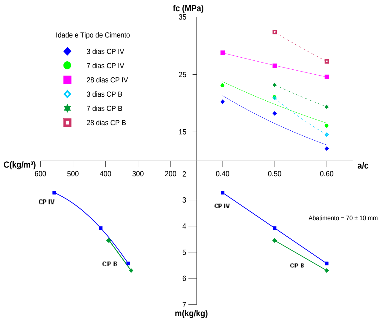
Figura 3 – Resistência à compressão média dos concretos conforme relação a/c
