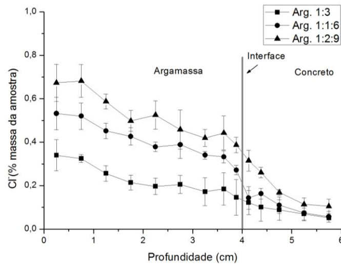
Figura 7 - Perfis de cloretos obtidos por meio de ensaio de imersão e secagem para os CPs moldados com 4,0 cm de revestimento de argamassa
