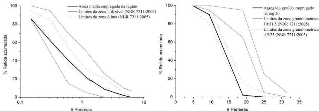
Figura 2 - Curvas granulométricas dos agregados miúdo e grúdo
