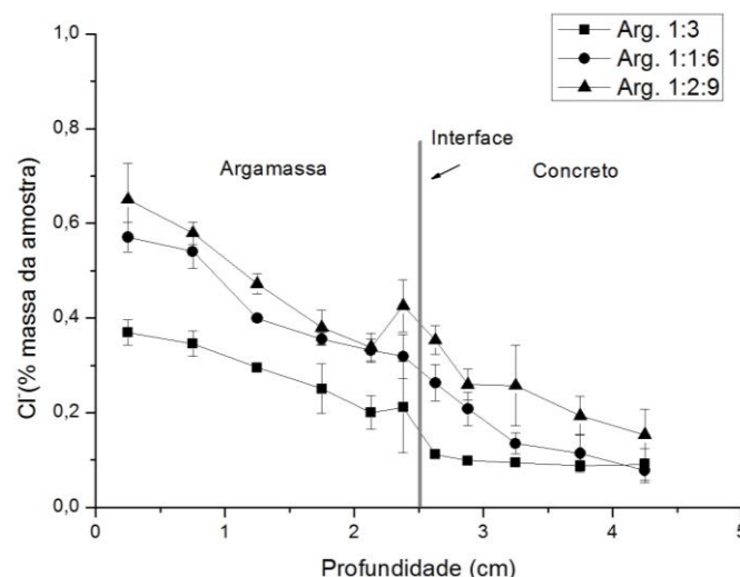
Figura 6 - Perfis de cloretos obtidos mediante ensaio de imersão e secagem para os CPs moldados com 2,5 cm de revestimento de argamassa
