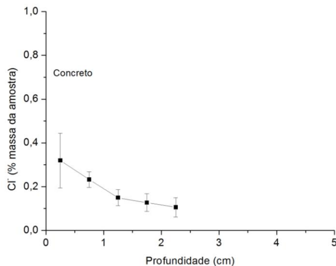
Figura 8 - Perfil de cloretos obtido por meio do ensaio de imersão e secagem para os CPs de referência moldados em concreto
