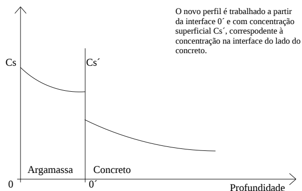
Figura 10 - Reescalonamento empregado para os perfis de cloretos no concreto
