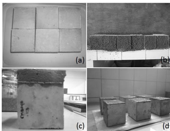
Figura 4 - (a) CPs limpos; (b) Chapisco aplicado; (c) CPs revestido com argamassa; e (d) Pintura epóxi aplicada
