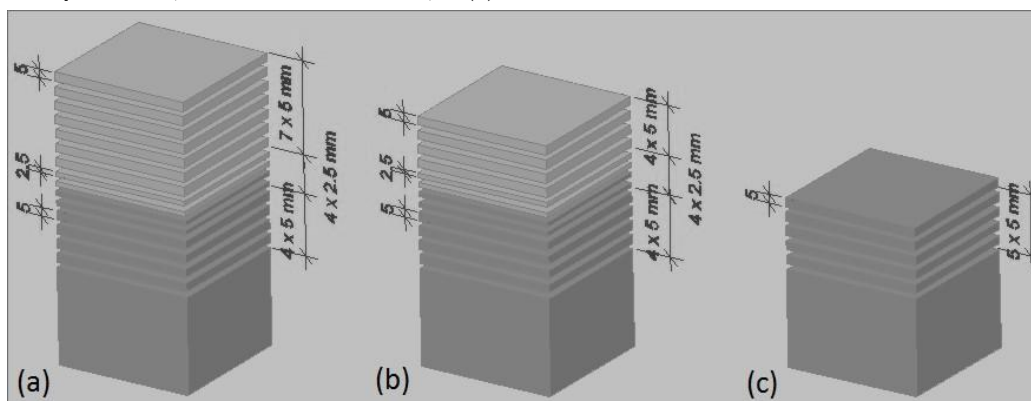
Figura 5 - Esquema da distribuição dos cortes: (a) Sistema duplo com 4,0 cm de revestimento; (b) Sistema duplo com 2,5 cm de revestimento; e (c) CPs de referência em concreto
