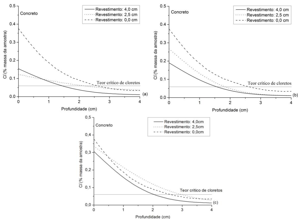
Figura 11 - Perfis de cloretos ajustados na zona do concreto, para as argamassas (a) 1:3, (b) 1:1:6 e (c) 1:2:9
