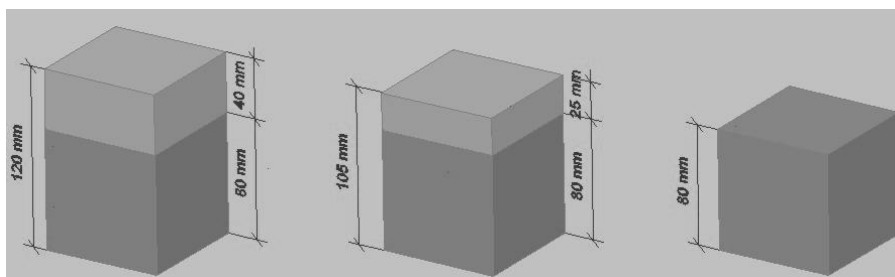
Figura 3 - Tipologias dos corpos de prova empregados na pesquisa com revestimento de 40 mm, 25 mm e sem revestimento
