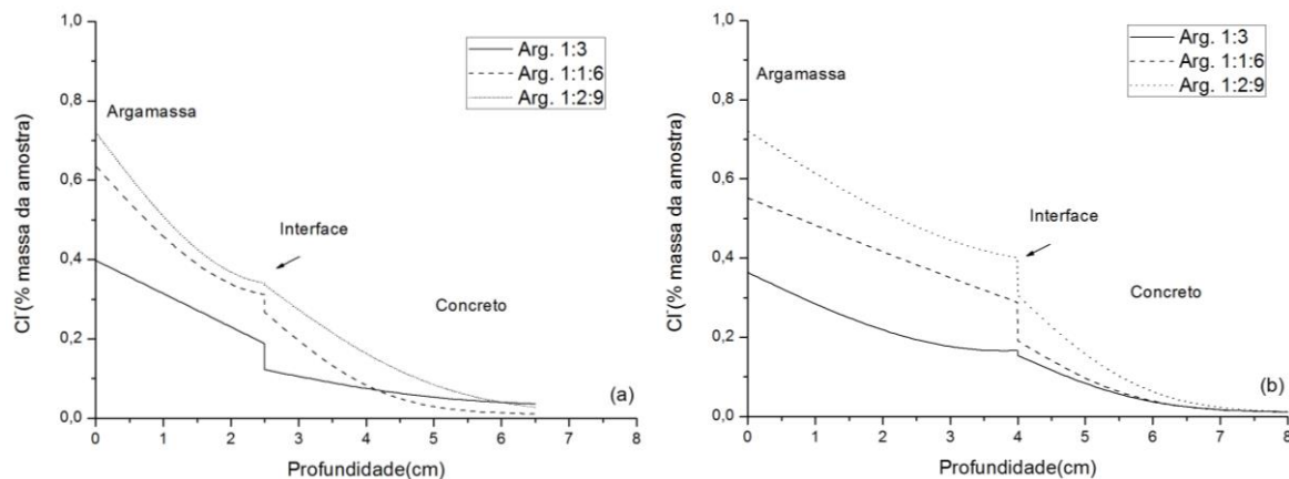
Figura 12 - Perfis ajustados para as espessuras de revestimento de (a) 2,5 cm e (b) 4,0 cm
