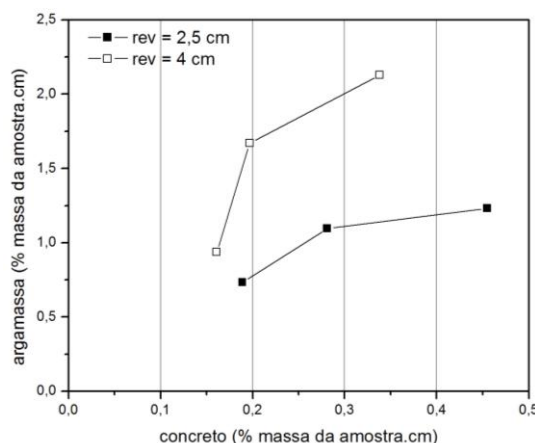
Figura 9 - Relação entre o acúmulo de cloretos na argamassa e no concreto
