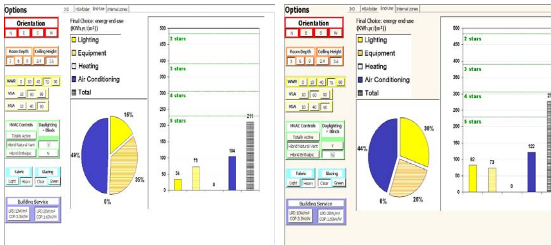
Figura 12 - Comparação de consumo de energia por uso final para dois casos: com e sem uso de iluminação natural
