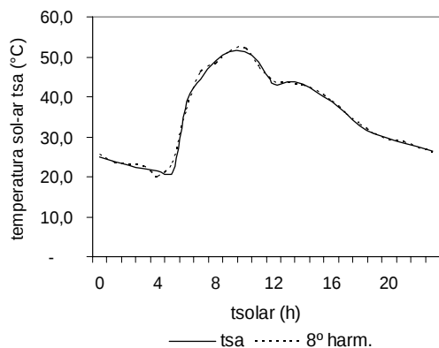
Figura 2 - Convergência da temperatura sol-ar para a parede com orientação leste, para o dia típico de verão de Campinas, SP, absorvância à radiação solar \alpha=0,61
