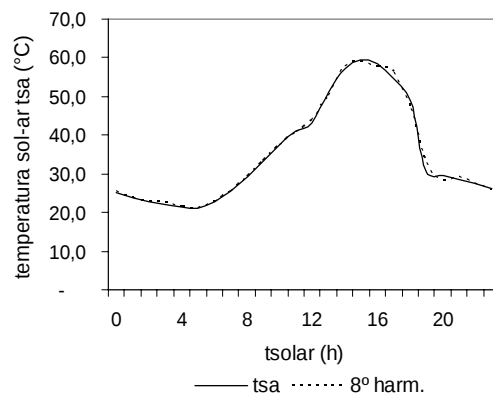
Figura 3: Convergência da temperatura sol-ar para a parede com orientação oeste, para o dia típico de verão de Campinas, SP, absorvância à radiação solar \alpha=0,61
