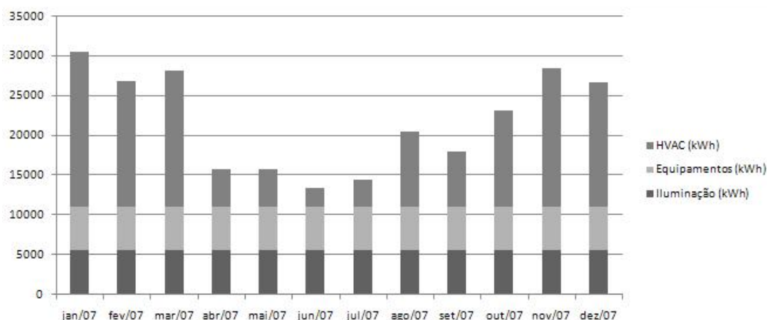
Figura 10 – Consumo de energia elétrica por uso final de uma agência bancária típica, localizada na ZB-3, Região Sul do Brasil
