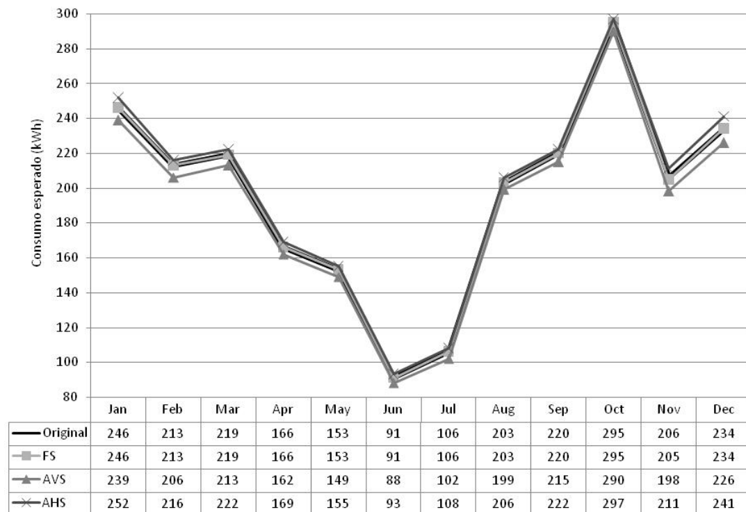
Figura 14 - Potencial de economia de energia elétrica do sistema de ar condicionado, considerando o projeto original e o projeto com as alterações propostas de FS, AVS e AHS, para a implantação da agência com a fachada principal para o leste na cidade de Cuiabá/MT, localizada na ZB-7 - consumo mensal em kWh
