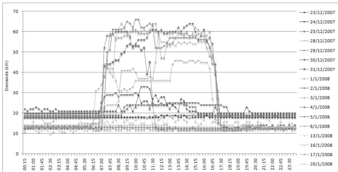
Figura 8 - Comportamento de carga diário de uma agência bancária típica, localizada na Região Sul do Brasil
