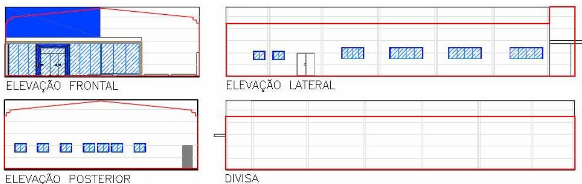
Figura 2 - Elevações do projeto padrão da agência bancária
