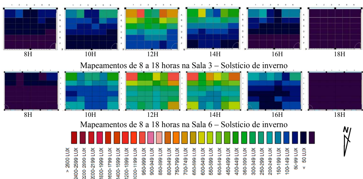
Figura 11 - Mapeamentos das salas da EEC, no solstício de inverno, com janelas abertas
