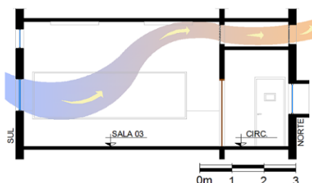
Figura 5 - Sistema de ventilação natural da Sala 3 da EEC
