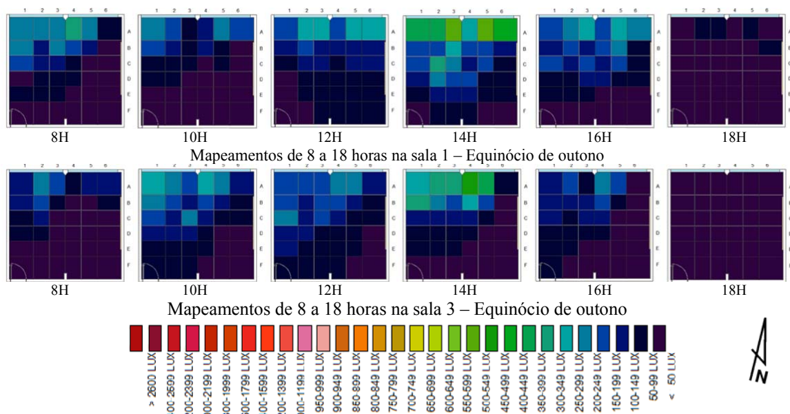
Figura 14 - Mapeamentos das salas da FAV, equinócio de outono
