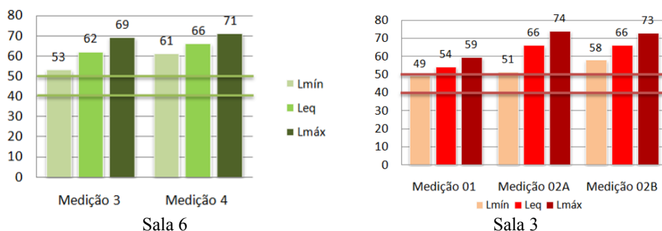
Figura 22 - Níveis de pressão sonora das medições realizadas nas salas da ECC
