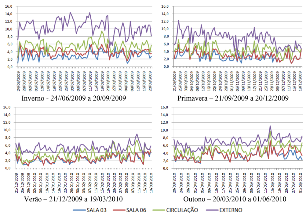
Figura 16 - Amplitudes térmicas diárias, por estação do ano, nas salas da EEC
