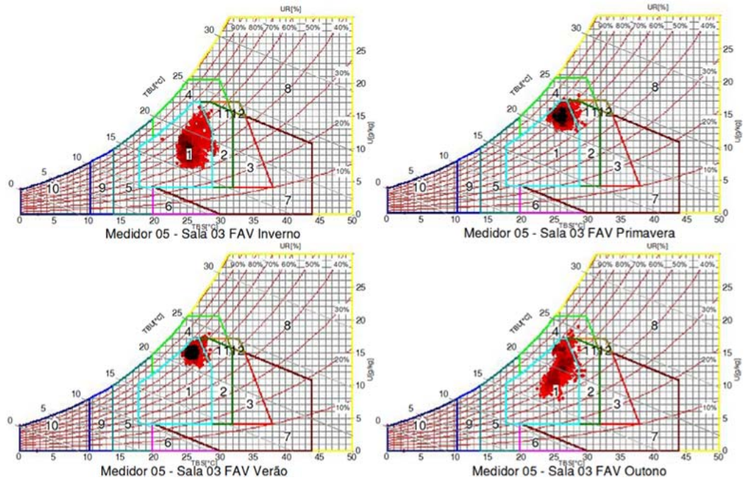
Figura 20 - Cartas psicrométricas, medidor 5, na sala 3, FAV
