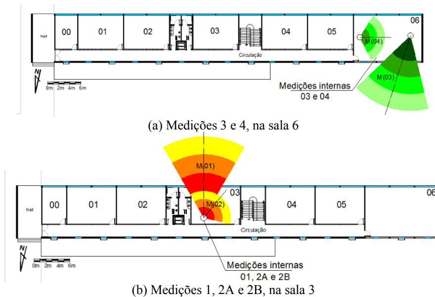
Figura 21 - Localização e direcionamento das medições nas salas da EEC
