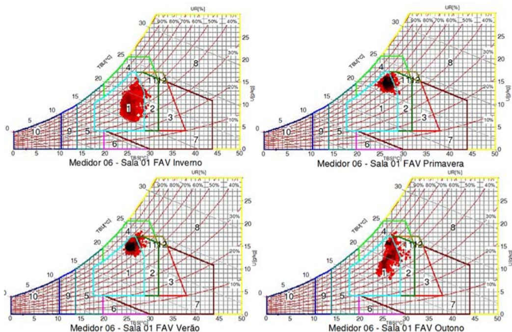
Figura 19 - Cartas psicrométricas, medidor 6, na sala 1, FAV
