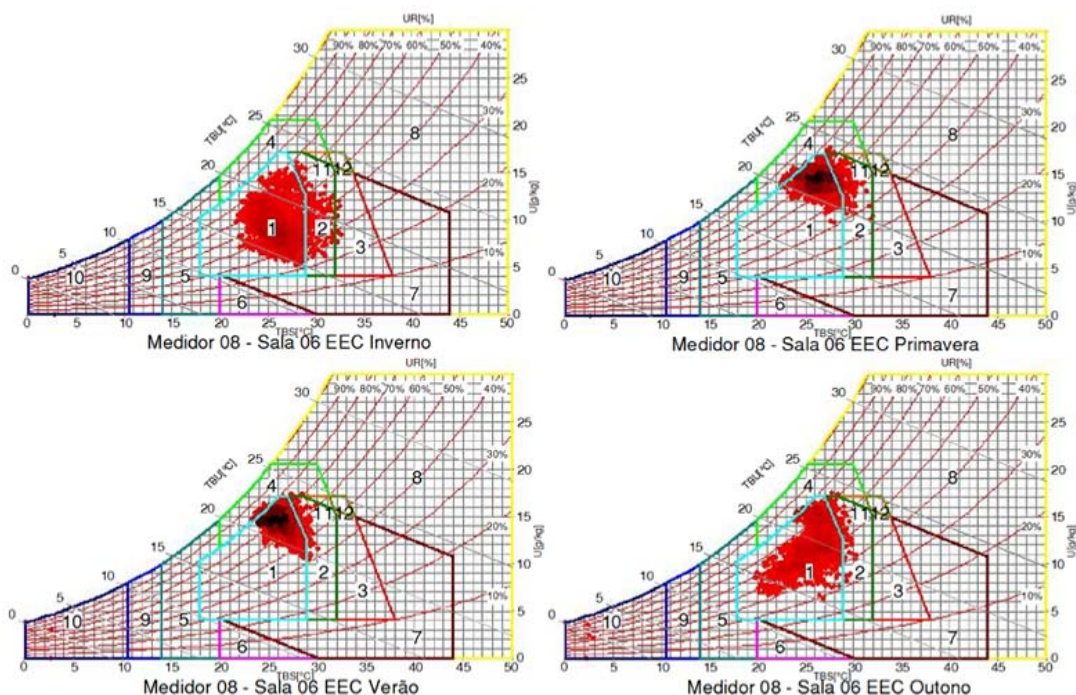
Figura 18 - Cartas psicrométricas relativas à sala 6, EEC
