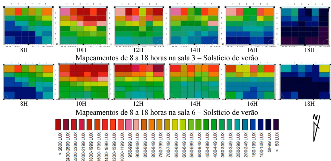
Figura 12 - Mapeamentos das salas da EEC no solstício de verão, com janelas abertas
