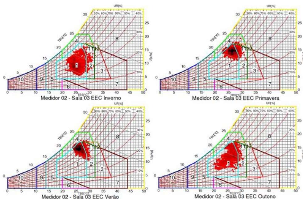
Figura 17 - Cartas psicrométricas relativas à sala 3, EEC
