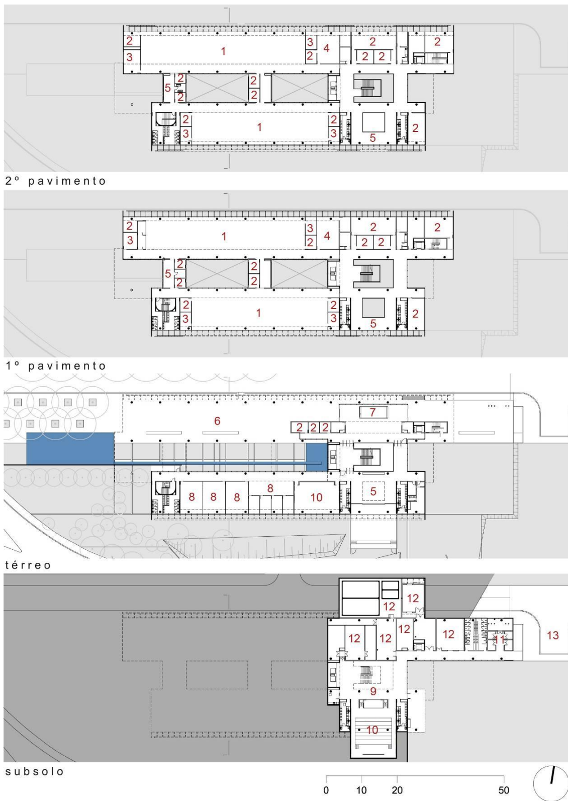
Figura 9 - SAP Labs Brazil, plantas dos pavimentos, escala 1/1.000
