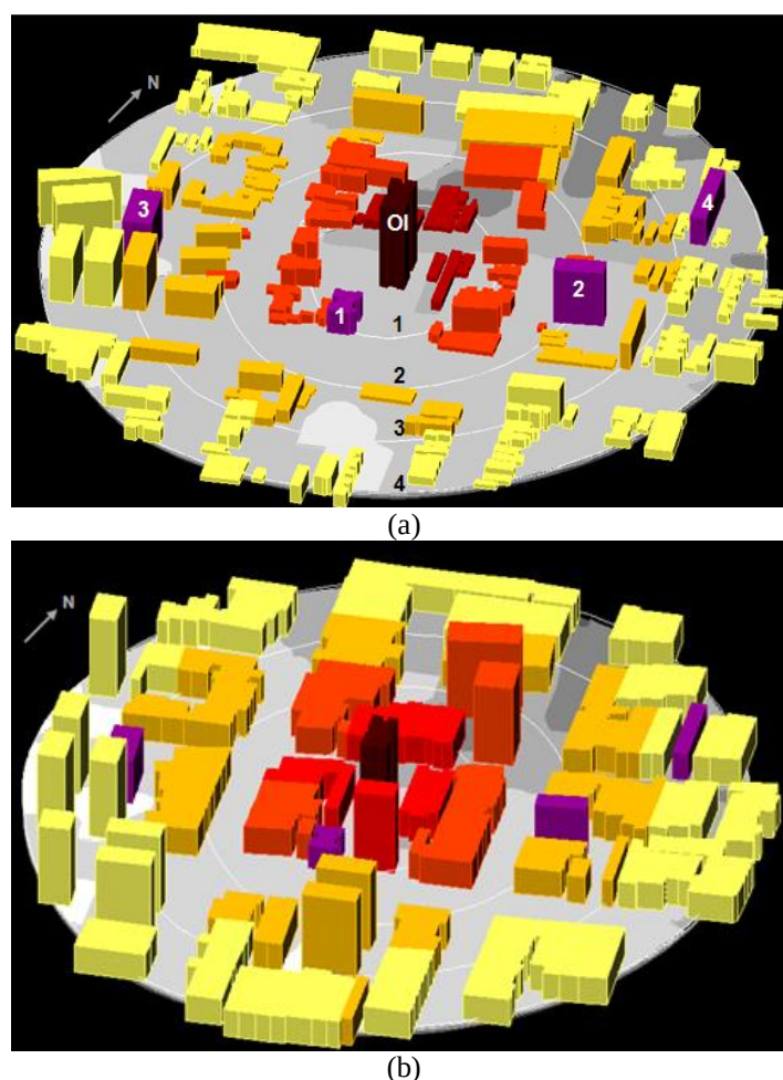
Figura 5 - (a) Cenário urbano real e (b) máximo de ocupação pelo plano diretor vigente
