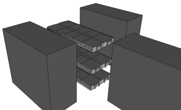
Figura 4 - Edifício real modelado com sombreamento do entorno e proteções solares - vista NE
