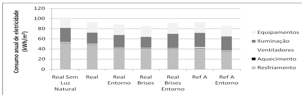
Figura 5 - Usos finais dos modelos simulados
