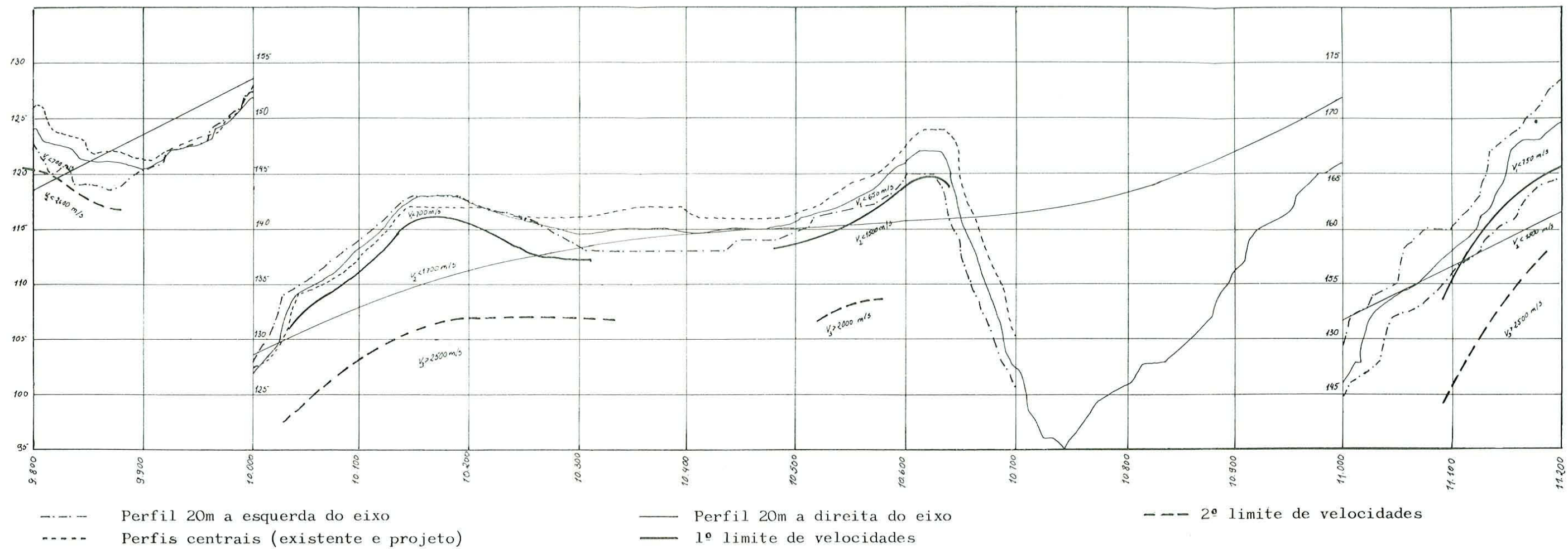
FIG. 3 - LIMITES DE VELOCIDADE SÍSMICAS REFERIDOS AO PERFIL CENTRAL (km 9,800 a 11,200)
