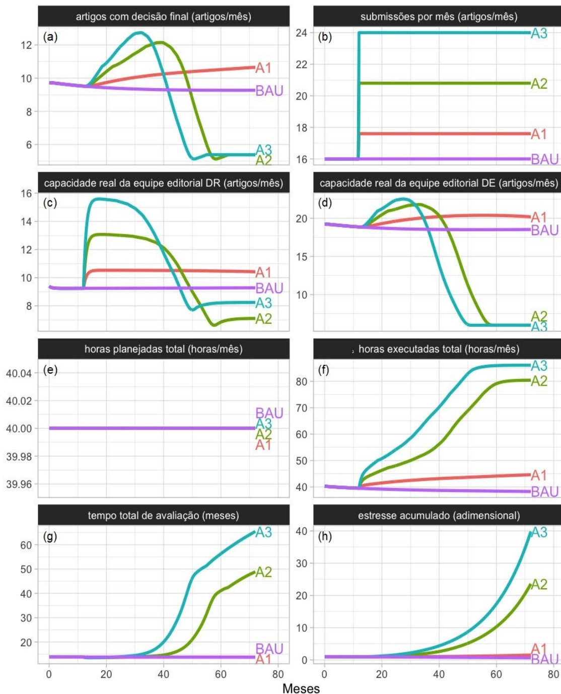
Figura 7 - Comportamento das variáveis nos cenários simulados
