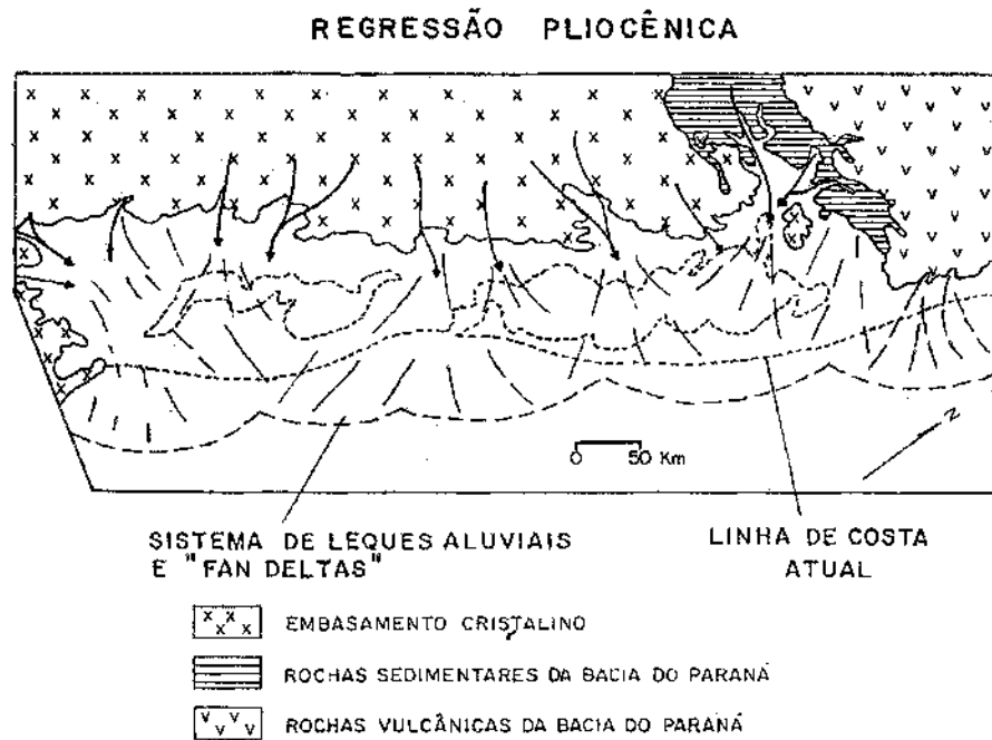
FIGURA 5 – EVOLUÇÃO PALEOGRÁFICA DA PLANÍCIE LITORÂNEA – RS, SEGUNDO VILLWOCK e TOMAZELLI, 1995.
