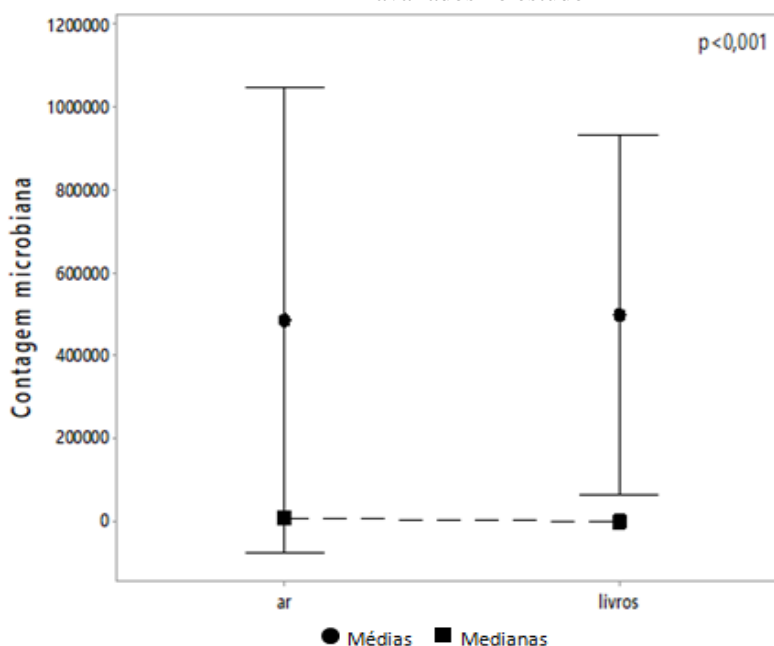
Gráfico 2 - Intervalos de confiança (95%) para a contagem microbiana (UFC) do ar e dos livros avaliados no estudo
