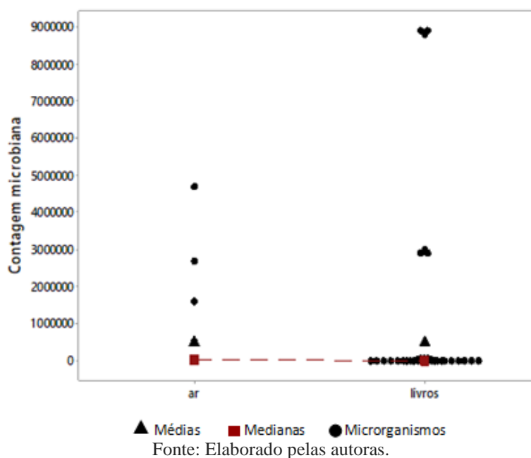
Gráfico 3 - Valores individuais da contagem microbiana (UFC) do ar e dos livros avaliados no estudo
