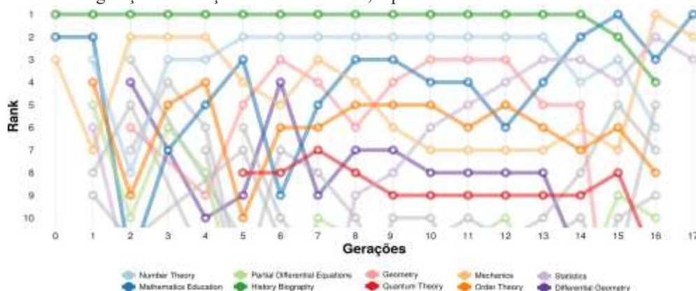
Figura 2 - Ranking dos tópicos do MSC, representado no eixo vertical, identificados em cada geração de atuação dos matemáticos, representadas no eixo horizontal
