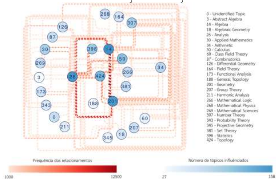
Figura 4 - Grafo de tópicos do conhecimento onde os vértices representam os tópicos identificados e as arestas representam a relação de influência
