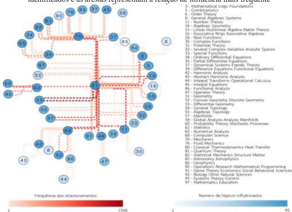
Figura 3 - Grafo de tópicos do conhecimento onde os vértices representam os tópicos identificados e as arestas representam a relação de influência mais frequente
