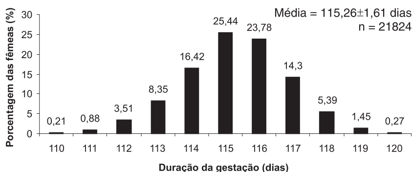
Figura 1. Frequência de distribuição da duração da gestação de suínos da genética Agroceres PIC®, em uma granja localizada no centro-oeste brasileiro no período de 2002 a 2003.
